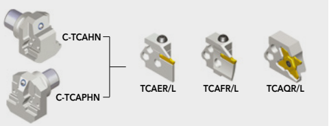
Système C-Adapter et HSK-T
