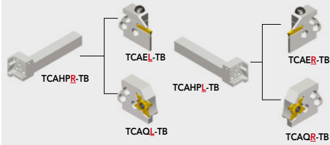
Système perpendiculaire avec canaux de lubrification interne Haute Pression
