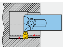
Utilisation rationnelle des flancs
